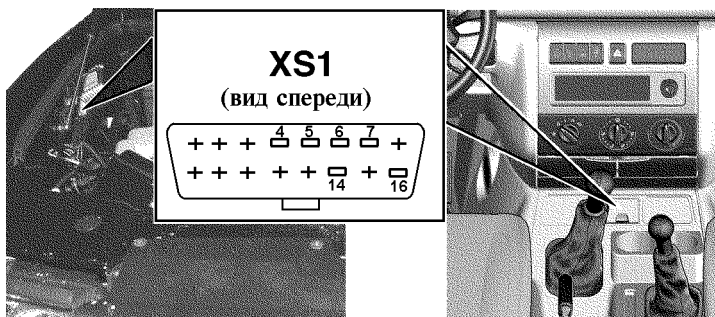
Рис. 9.21. Диагностический разъем (XS1): 4, 5 -масса; 6, 14 -Сап-линия; 7 -К-линия; 16 -+12В
