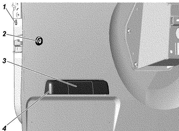
Рис. 3.18. Дверь задка: 1 -рычаг блокировки внутренней ручки открывания двери; 2 -замок; 3 -подвижная часть ручки двери; 4 -корпус ручки двери
