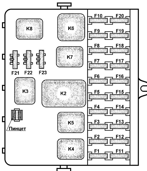
Рис. 9.37. Монтажный блок:
