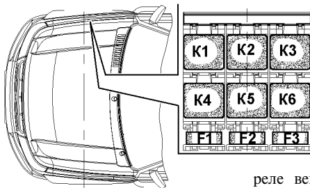
Рис. 9.39. Реле и предохранители:
