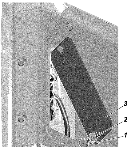
Рис. 9.37. Люк доступа к задним фонарям: 1 -фиксатор держателя крышки; 2 -держатель крышки; 3 -крышка
