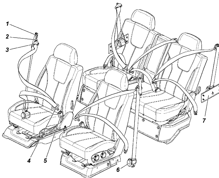
Рис. 3.25. Ремни безопасности:
